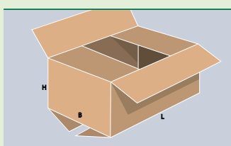
Faltkarton FEFCO 0201 mit zusammenstoßenden Boden-Deckel-Klappen
